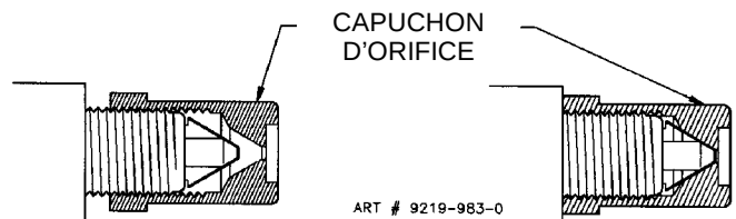
FIGURE 15C RÉGLAGE POUR GAZ NATUREL
