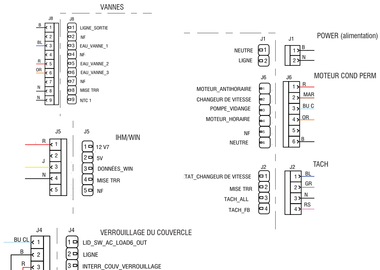
Illustration 5 – Broches et connecteurs
