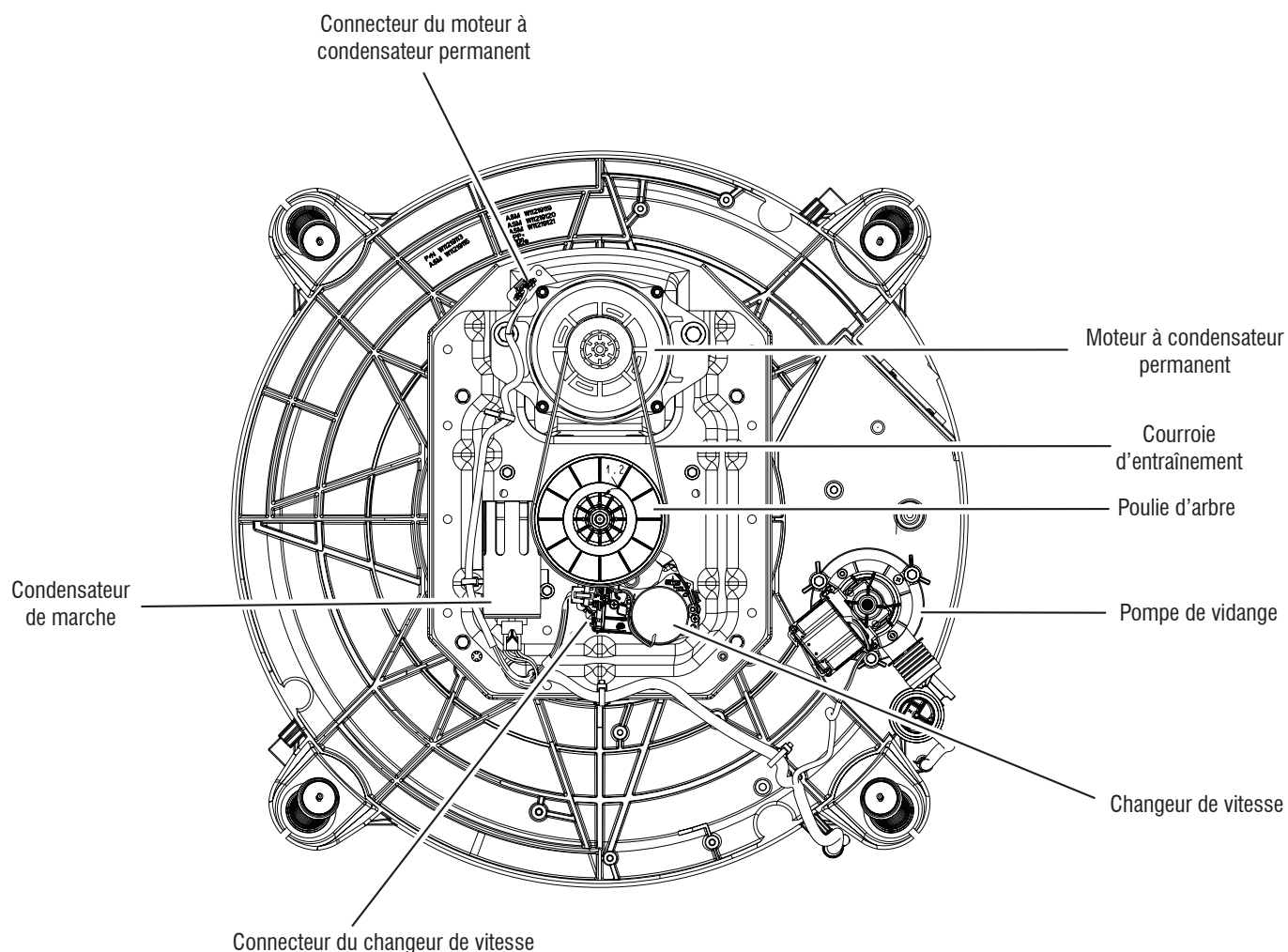
Illustration 8 – Vue du bas – COND PERM
