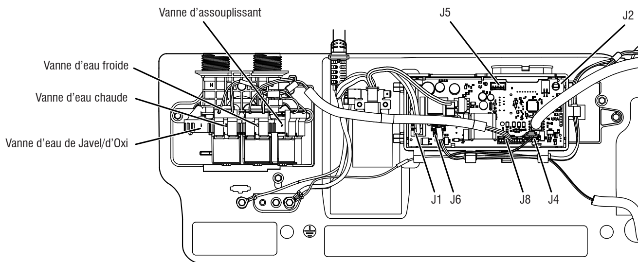
Illustration 7 – Module de commande principal (MCA)
