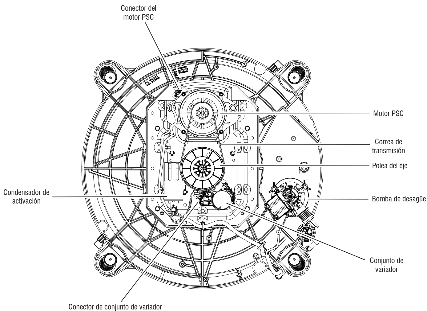
Figura 8: Vista inferior, PSC
